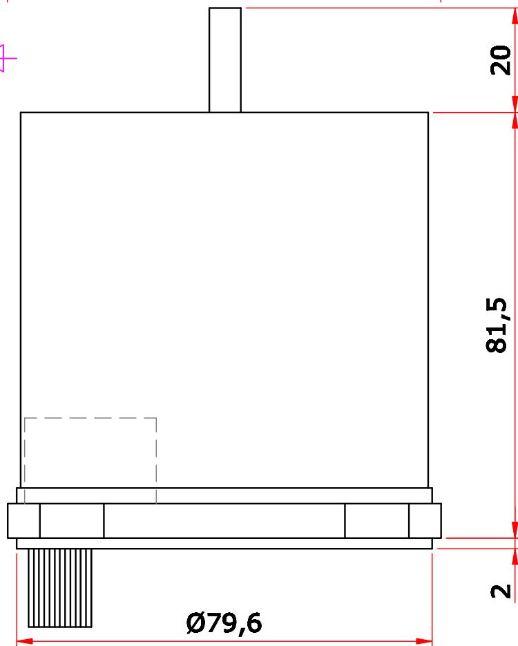
Einbaumaße 4 FGH 10 - 432 Mounting dimensions 4 FGH 10 - 432
